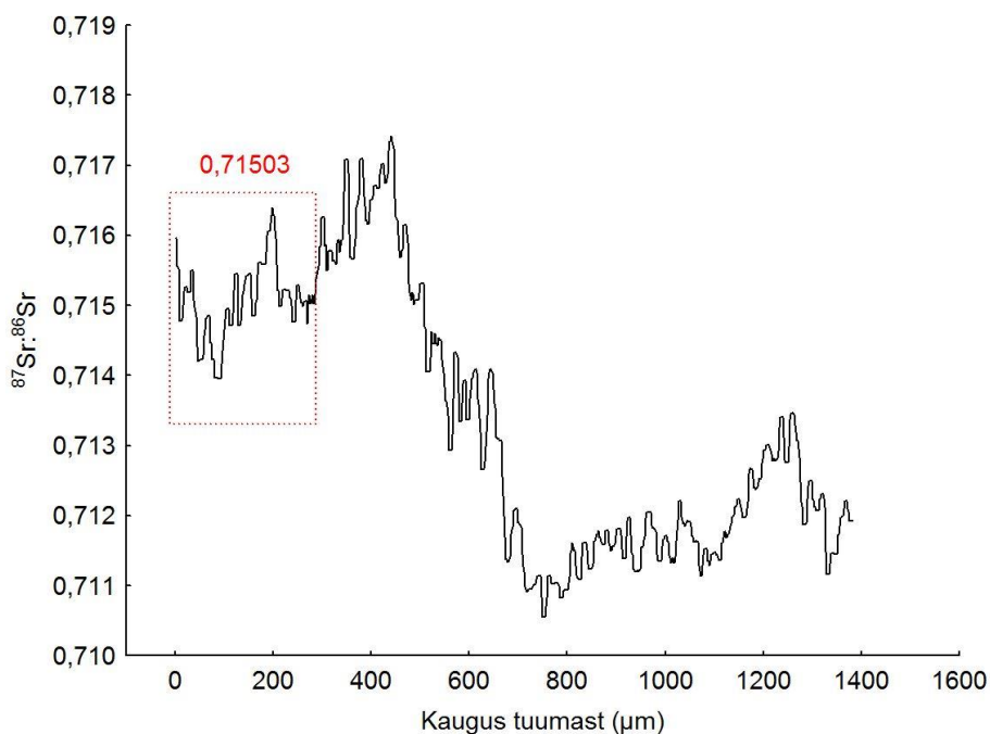
Joonis 5. Emajõeest Praagalt 03.05.2018 püütud asustatud tõugja otoliidi ^{87}\text{Sr}:^{86}\text{Sr} profiil (TL=69 cm, suguküps emane). Punase punktiirjoonega on tähistatud profiili osa, kust arvutati keskmine koorumisjärgne ^{87}\text{Sr}:^{86}\text{Sr} näit. Vaata ka jooniselt 6 sama kala otoliidi Sr:Ca ja Ba:Ca profiili.
