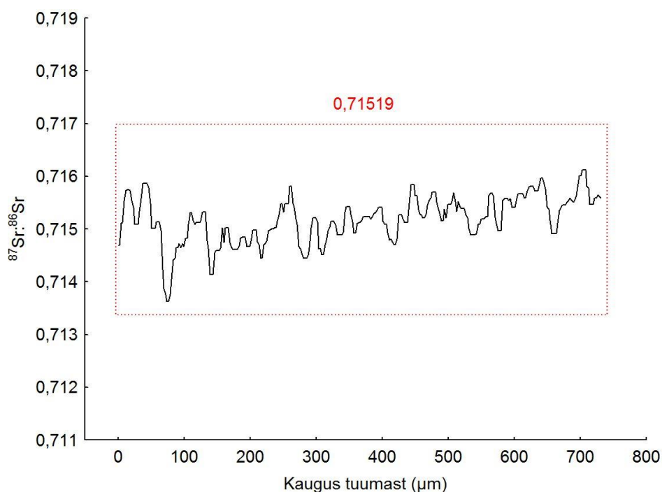
Joonis 1. Haaslava kalamajandist 17.08.2011 kogutud ühesuvisel tõugja otoliidi ^{87}\text{Sr}:^{86}\text{Sr} profiil. Punase punktiirjoonega on tähistatud profiili osa, kust arvutati keskmine kooremisjärgne ^{87}\text{Sr}:^{86}\text{Sr} näit.
