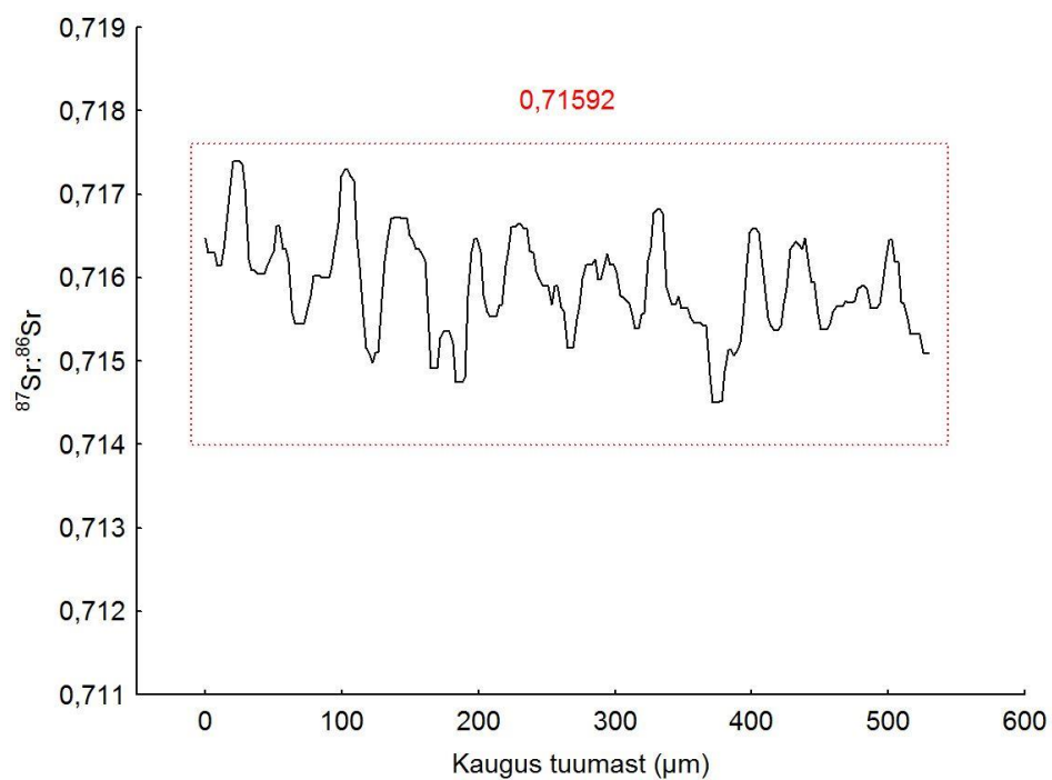
Joonis 3. Karisto ojast 29.08.2018 püütud kahestruise tõugja otoliidi ^{87}\text{Sr}:^{86}\text{Sr} profiil. Punase punktiirjoonega on tähistatud profiili osa, kust arvutati keskmine koorumisjärgne ^{87}\text{Sr}:^{86}\text{Sr} näit.
