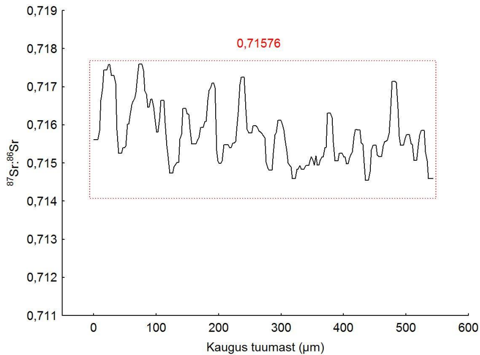
Joonis 2. Haaslava kalamajandist 21.09.2018 kogutud kahestruise tõugja otoliidi ^{87}\text{Sr}:^{86}\text{Sr} profiil. Punase punktiirjoonega on tähistatud profiili osa, kust arvutati keskmine koorumisjärgne ^{87}\text{Sr}:^{86}\text{Sr} näit.
